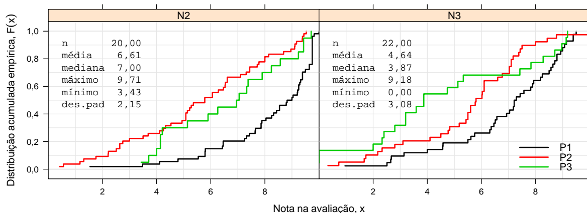
Figura 1: Distribuição acumulada empírica das notas dos alunos nas três avaliações de Estatística Básica. Estatísticas descritivas são fornecidas dentro do gráfico para as notas da terceira prova.
