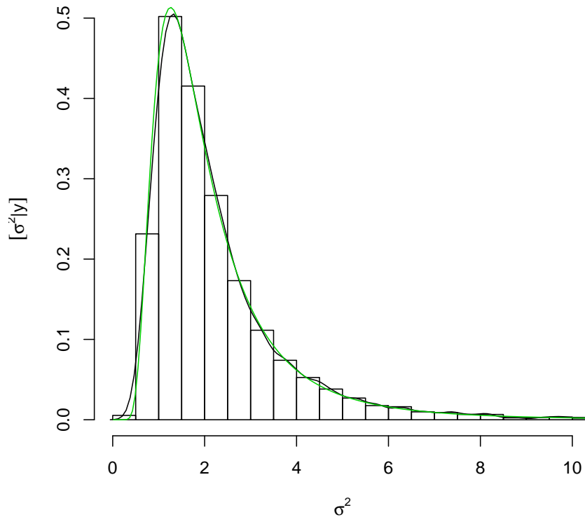
Figura 3: Histograma e densidade estimada das amostras da posteriori comparados com a expressão analítica da posteriori.
